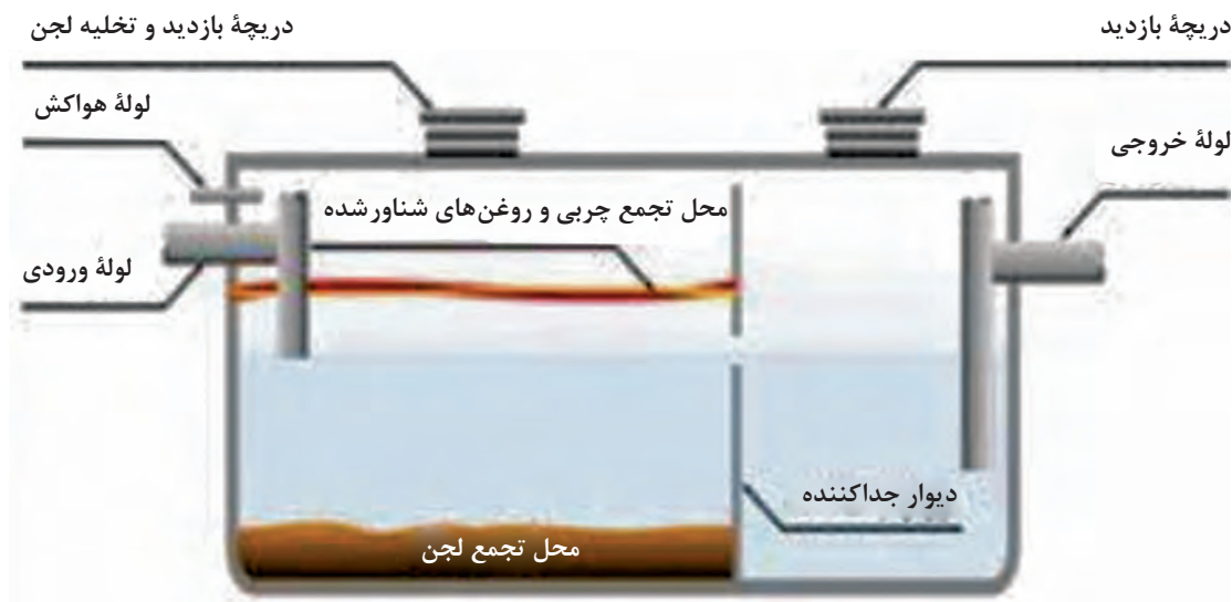
شکل ۱۴- سپتیک تانک
