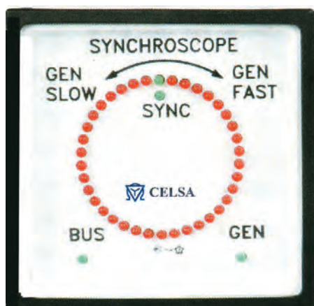
شکل ۲۰- سنکروسکوپ و مدار یک سنکروسکوپ ساده
