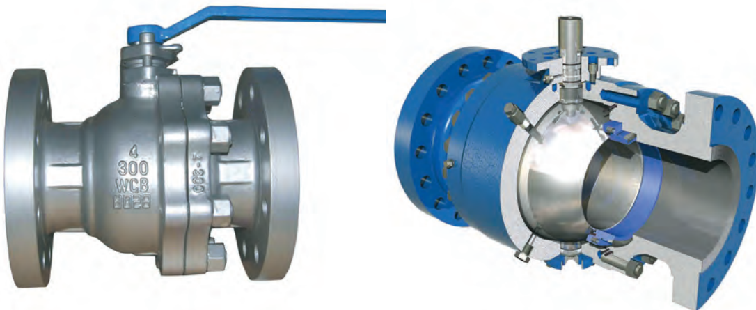
شکل ۵۳– شیر گُروی
