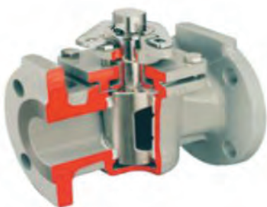
شکل ۴۸- شیر سماوری
