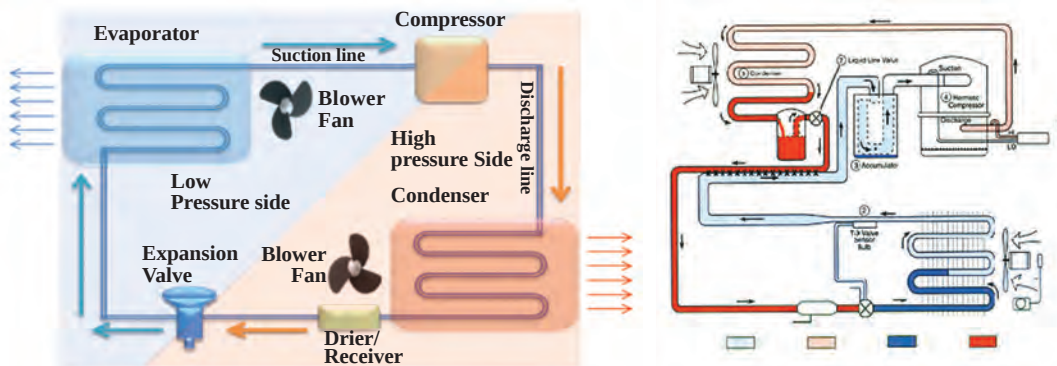
شکل ۲۹- سیستم انجماد (تبرید)
