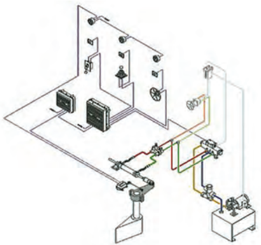
شکل ۲۷- سیستم سکان
