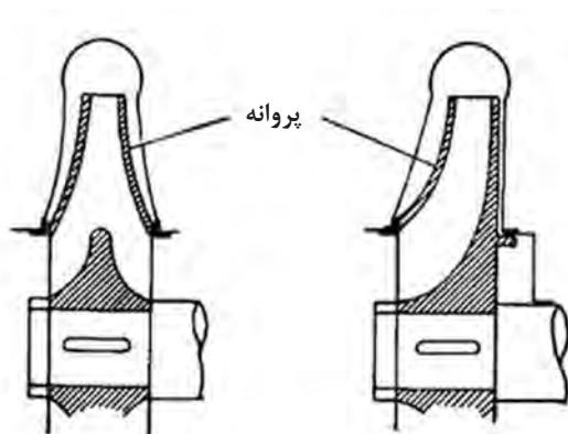
پروانه دو مکشه
