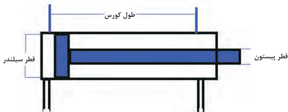
شکل ۱۷- مشخصات فنی و هندسی سیلندره‌ای هیدرولیک
